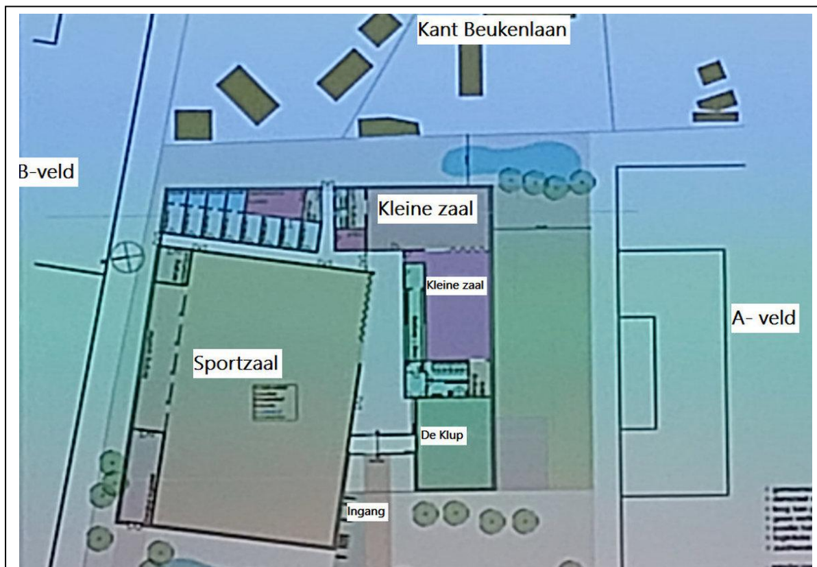
Figuur 56 De schets van het grondplan van de nieuwe sporthal
